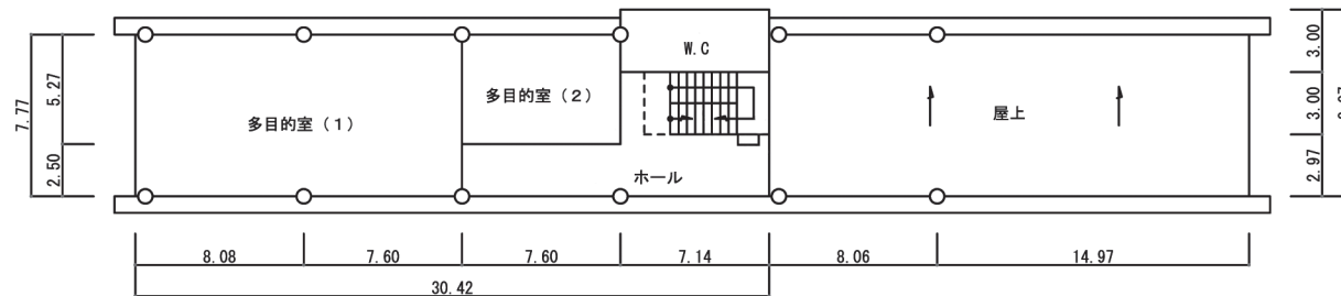
本館 3階
