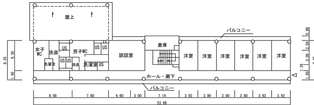
本館 2階
