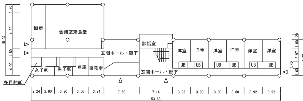
本館 1階
