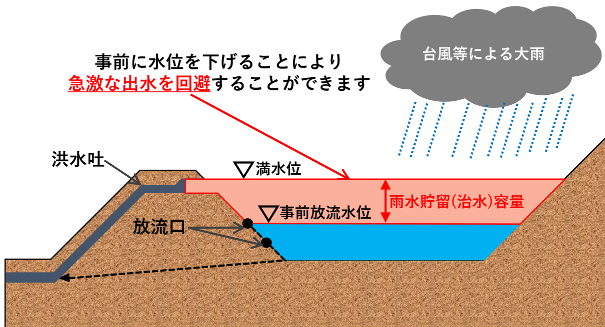
※ため池の低水位管理のイメージ
